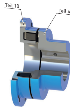
Bauart E
